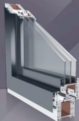
MyUnity CANTO Flügel flächenversetzt
