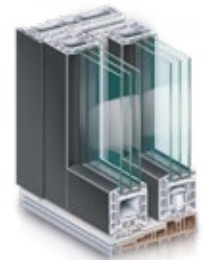
Hebe-Schiebe-Tür Kunststoff-Alu PremiDoor 80 und PremiDoor 95
