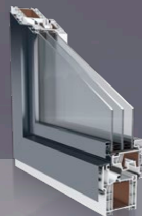
MyUnity CONTUR Flügel halbflächenversetzt
