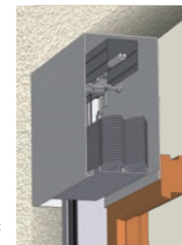
Raffstore-Bauelement mit sichtbarer Blende.
