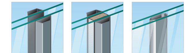
Standardklebesprossen
