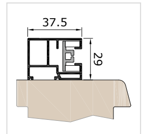
Führungsschiene FS Z37VP
