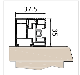
Führungsschiene FS Z37VP, Putzvariante
