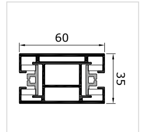
freitragende Kämpferschiene FS ZT60V
